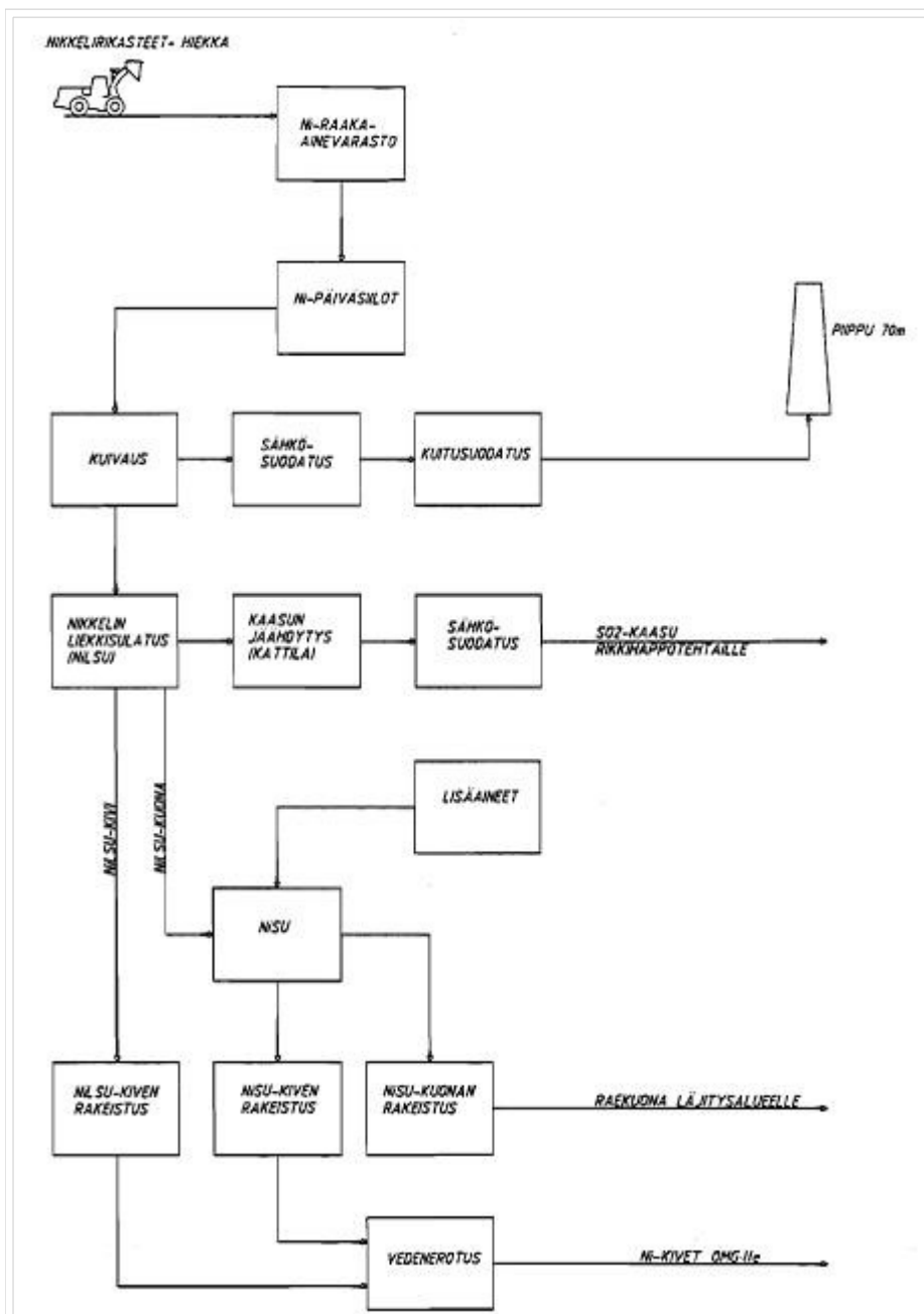
Kuva 23.2 Nikkelin sulatuksen prosessikaavio. (Outokumpu Harjavalta Metals Oy 2002). NSU = nikkelisähköuuni.
