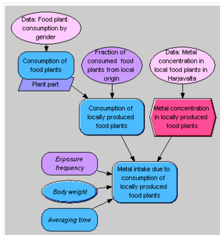
Kuva 7.4. Esimerkki syy-seurauskaaviosta.
