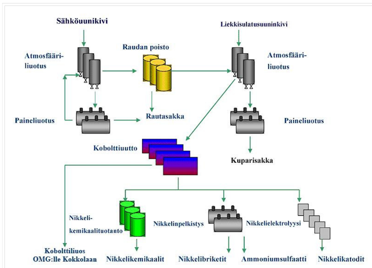
Kuva 23.3 Yleistetty prosessikaavio nikkeli tuotteiden valmistamisesta sähköuunin ja liekkisulatusuunin nikkelikivestä. Kuva: www.nornik.fi (13.3.2008).
